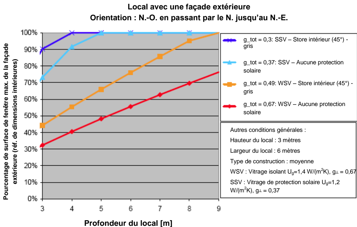
Figure 2 : Pourcentage de surface de fenêtre maximum de la façade extérieure pour un local d'une hauteur libre de 3 m et avec une façade extérieure orientée vers le nord pour différentes profondeurs de local et différentes valeurs de g_{tot}
