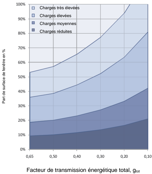
Figure 9 : Estimation du niveau des apports solaires d'une zone non conditionnée en fonction de la protection solaire et de la part de surface de fenêtre respectivement de la surface de fenêtre rapportée à la surface de plancher nette.
