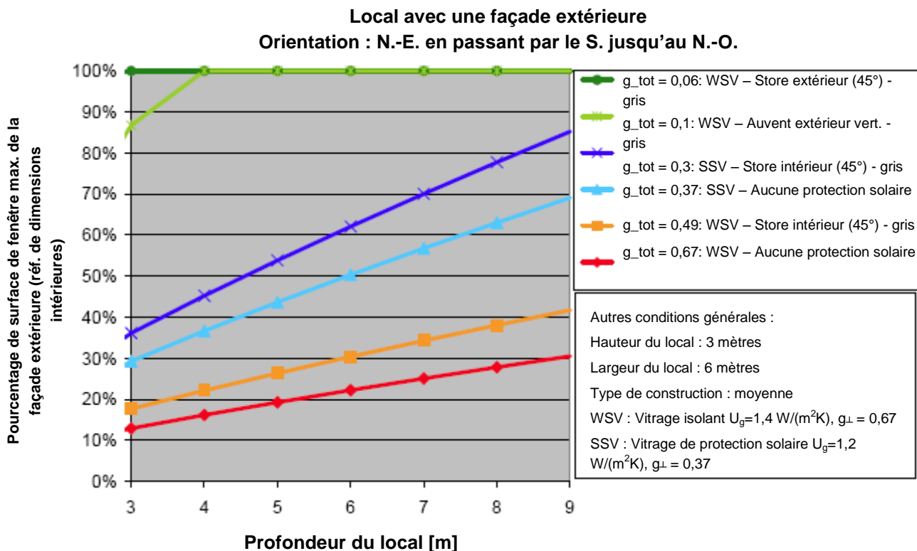
Figure 1 : Pourcentage de surface de fenêtre maximum de la façade extérieure pour un local d'une hauteur libre de 3 m et avec une façade extérieure orientée vers le nord-est en passant par le sud jusqu'au nord-ouest pour différentes profondeurs de local et différentes valeurs de g_{tot}
