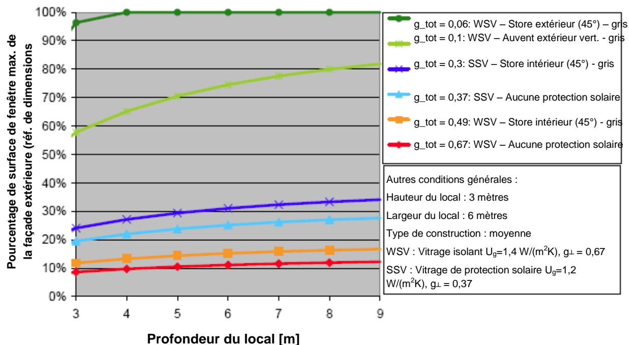
Figure 3 : Pourcentage de surface de fenêtre maximum de la façade extérieure pour un local d'une hauteur libre de 3 m et avec deux façades extérieures orientées vers le nord-est en passant par le sud jusqu'au nord-est pour différentes profondeurs de local et différentes valeurs de g_{tot} .
